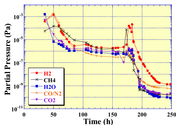
図4 : ベーキング中の残留ガス分析
