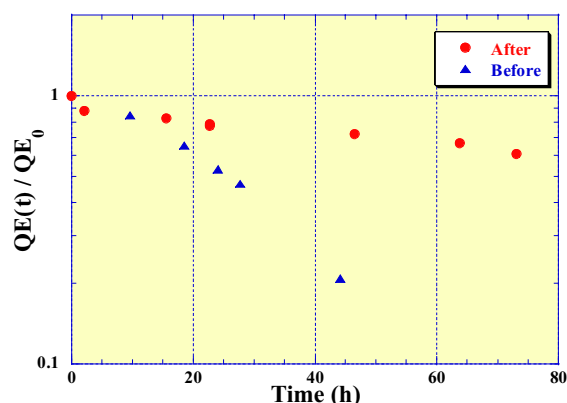
図5 : base-lifetime測定結果
