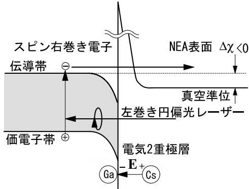
図1 : NEA表面からの電子放出
