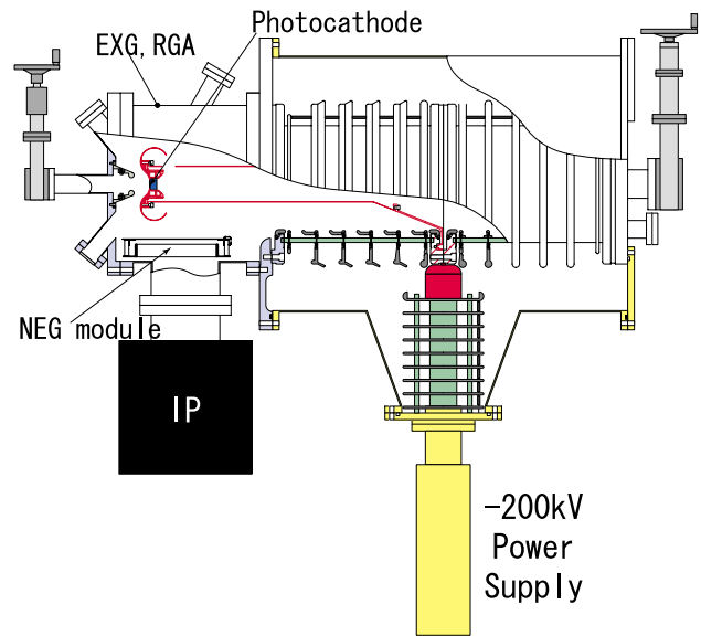
図2 : 200keV電子銃の断面模式図
