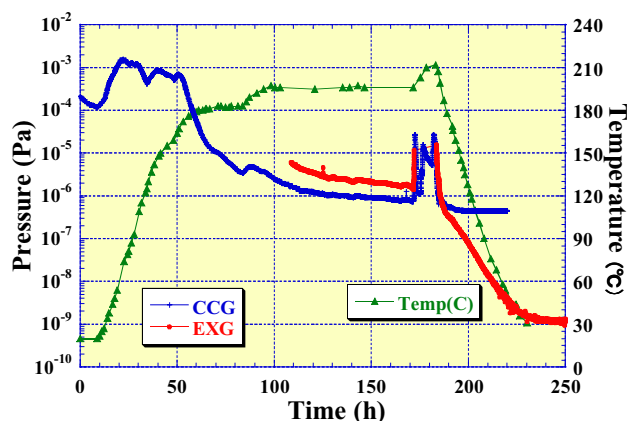
図3 : ベーキング中の真空度
