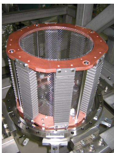
写真1 : NEGモジュール装着時の写真
