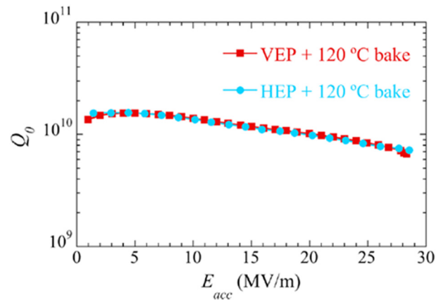
Figure 10: 縦型方式と横型方式で EP した同一の Nb 空洞の Q_0 - E_{acc} カーブ。文献[9]より。
