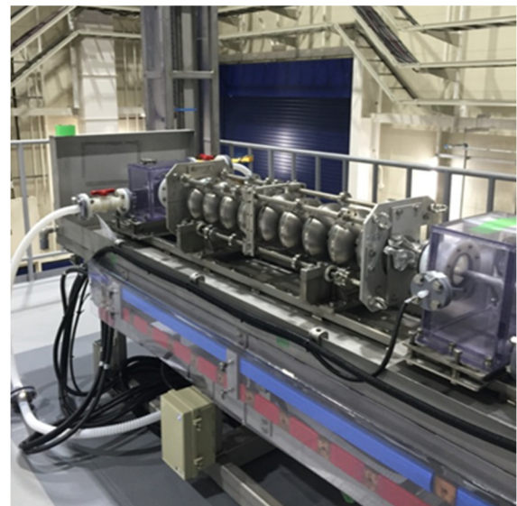
Figure 4: 空洞に治具と配管の取り付け.
