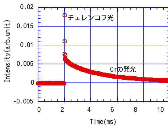
第5図 アルミナ蛍光板の減衰特性
