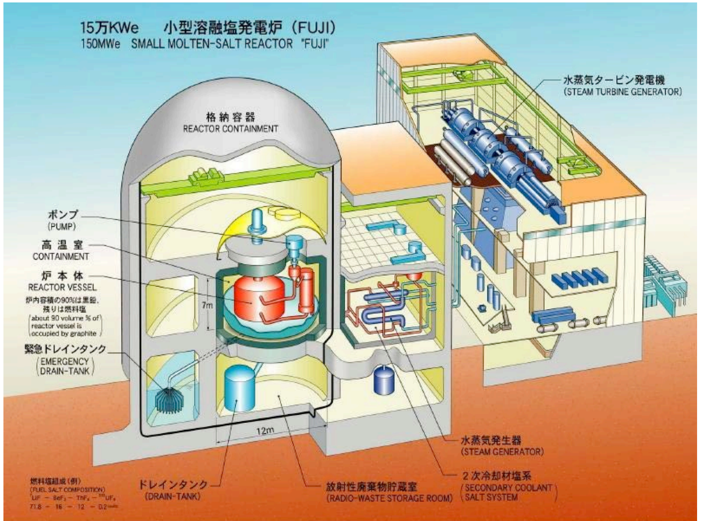
図3 小型熔融塩発電炉 FUJI の全体図
