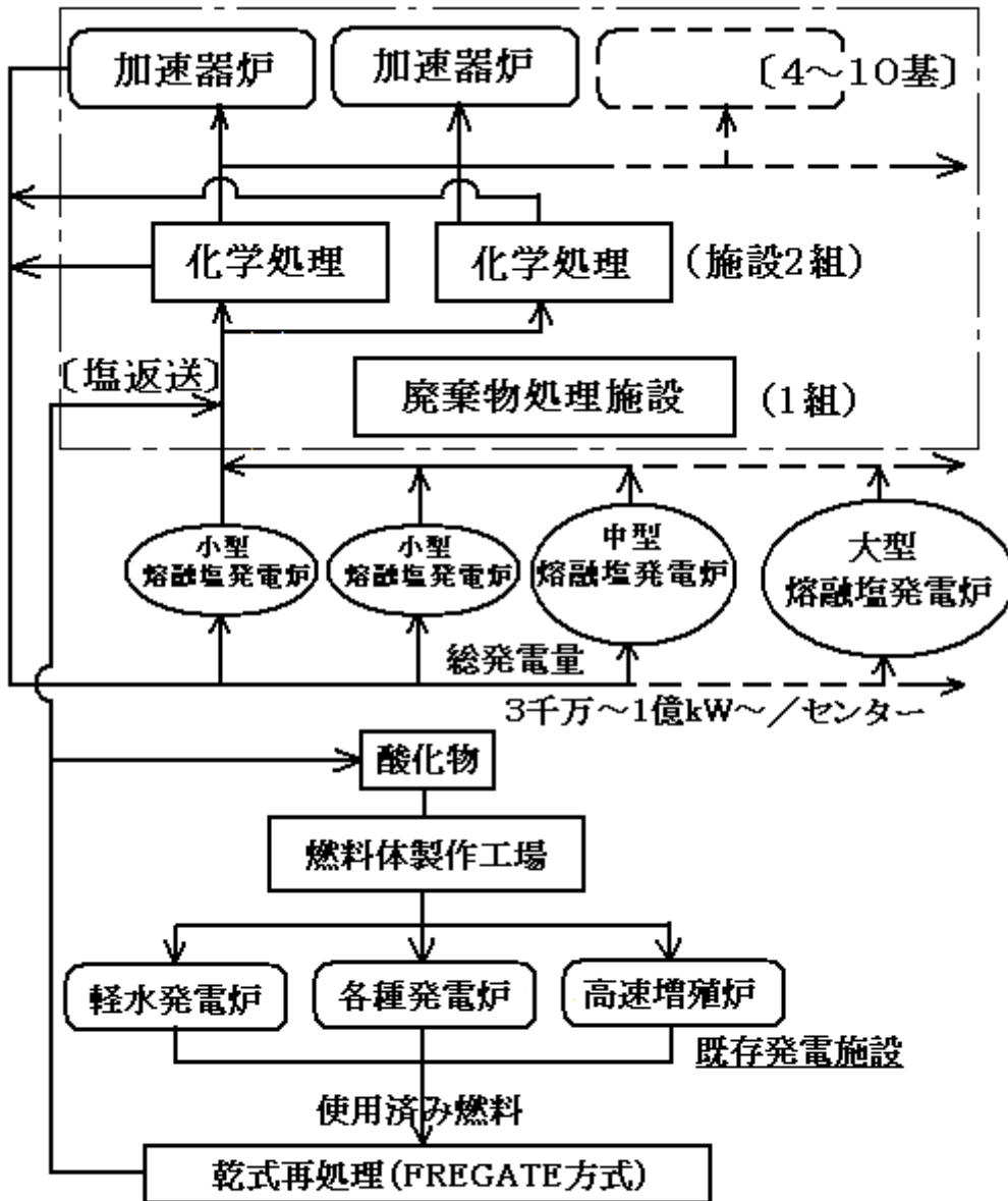
図6 加速器熔融塩増殖施設と熔融塩発電炉の組み合わせシステム〔トリウム熔融塩核エネルギー協働システム〕
