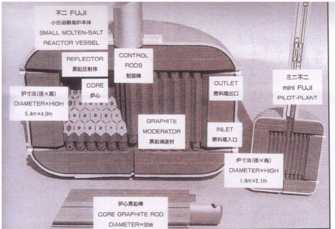
図2 小型熔融塩発電炉FUJIと超小型miniFUJI(右)の炉本体断面模型図
