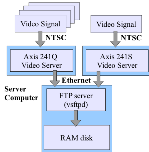
図 7: FTP 送信機能により画像ファイルをサーバーに連続的に送信する
