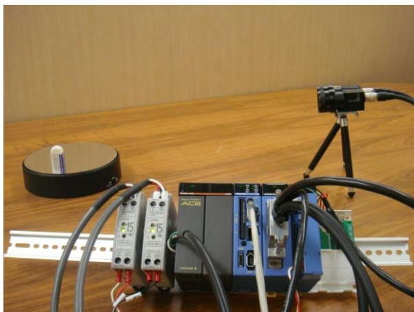
図 1 : 評価中の画像処理ユニット。左端の黒いモジュールは電源モジュール。その右隣が F3RP61。さらにその右隣が F3UM02。
