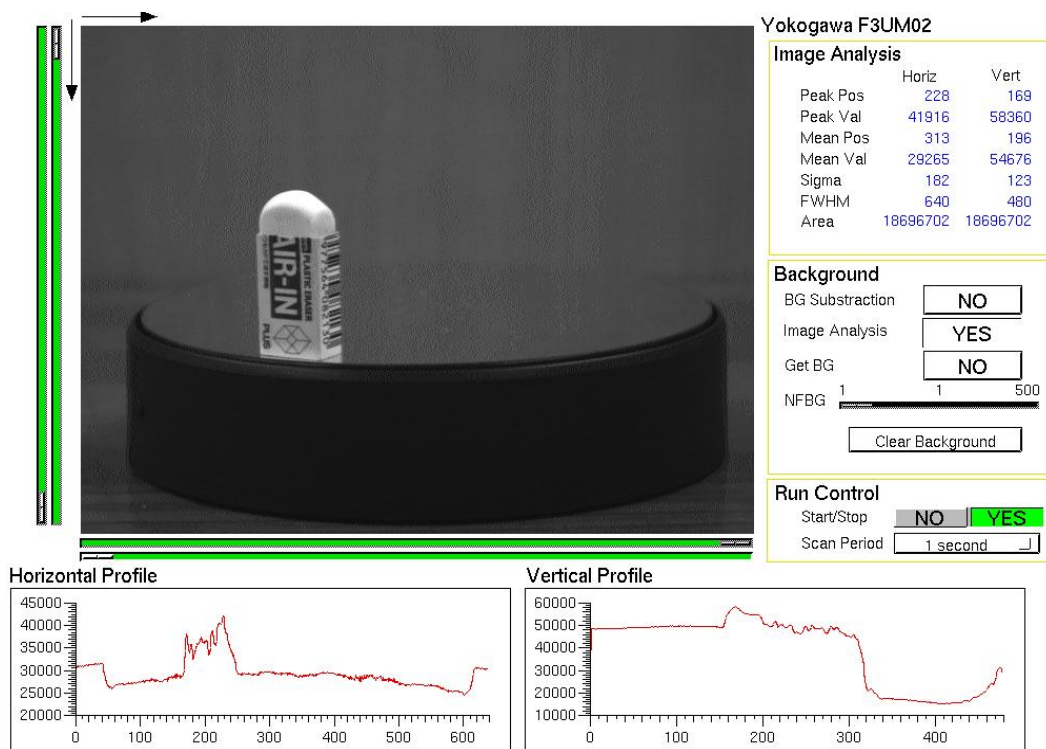
図 2 : EDM により作成された GUI。画像データの左と下に添えられたスライダーは Region of Interest (ROI) を graphicsRecord に設定するために使用される。その下の左側のグラフは水平方向へのプロジェクション、右側のグラフは鉛直方向へのプロジェクションを示す。プロジェクションの原点は画像の左側上端に採られている。
