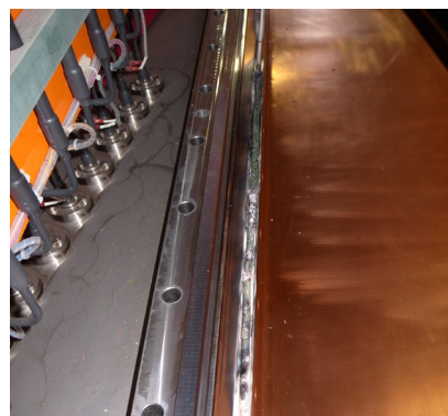
Figure 4: Burned-out C-ring in fRC-W resonator. 焦げた原因は接合面の締め付けが不十分であると考
