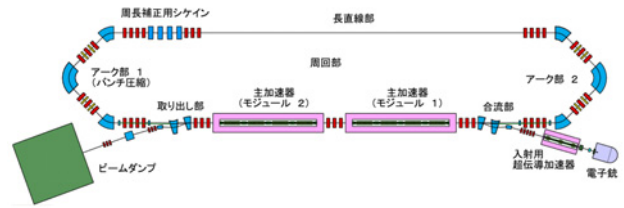
図4：コンパクトERLの機器配置。
